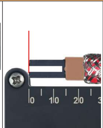
4 : Réglette graduée incorporée dans le couvercle, avec butée mécanique à 0 cm , pour faciliter la mesure de la longueur de dégainage.
